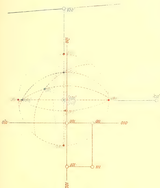
10. Альбитъ.
